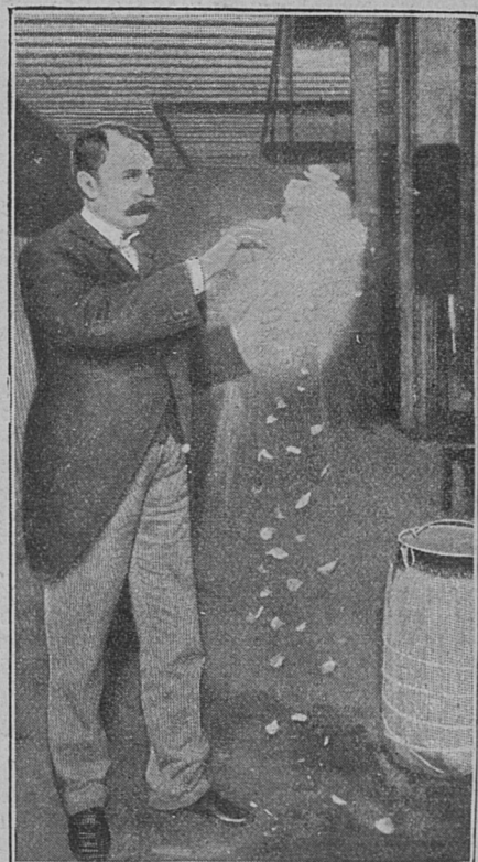
Распаденіе цвѣтовъ, погруженныхъ въ жидкій воздухъ.
